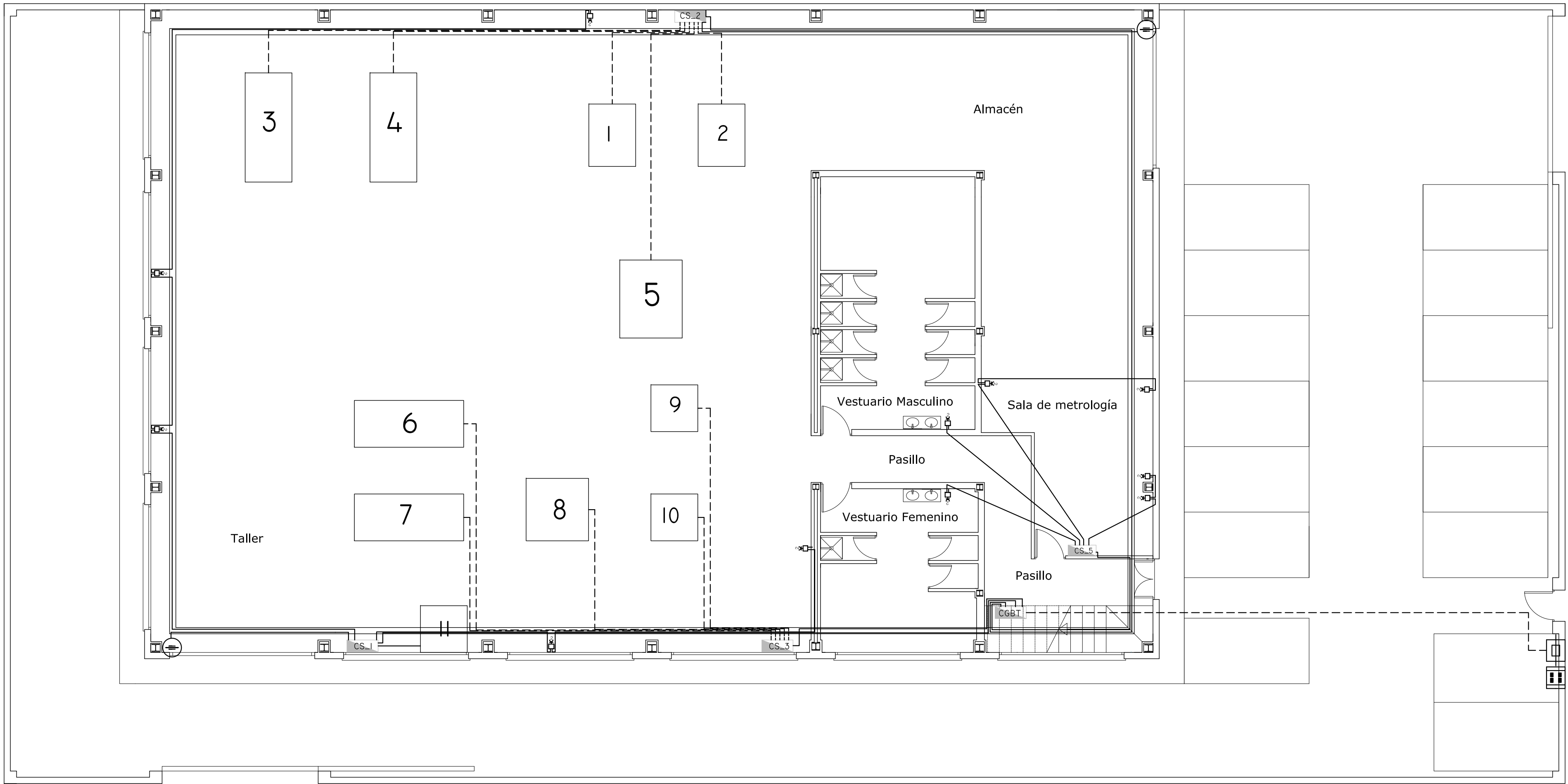
PLANTA BAJA
