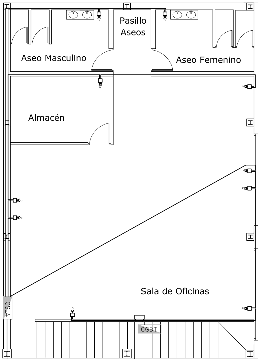
PLANTA PRIMERA
