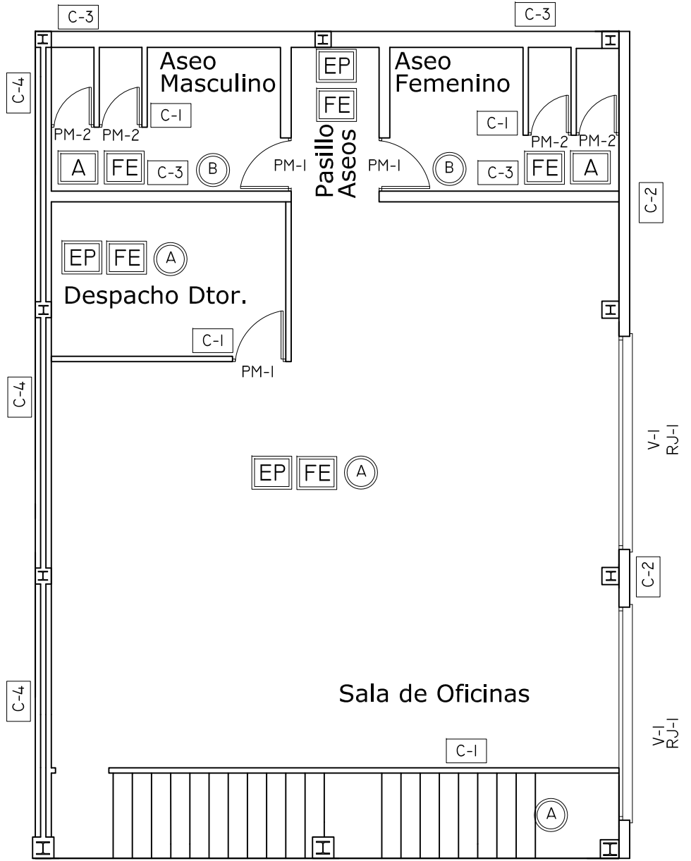
PLANTA PRIMERA
