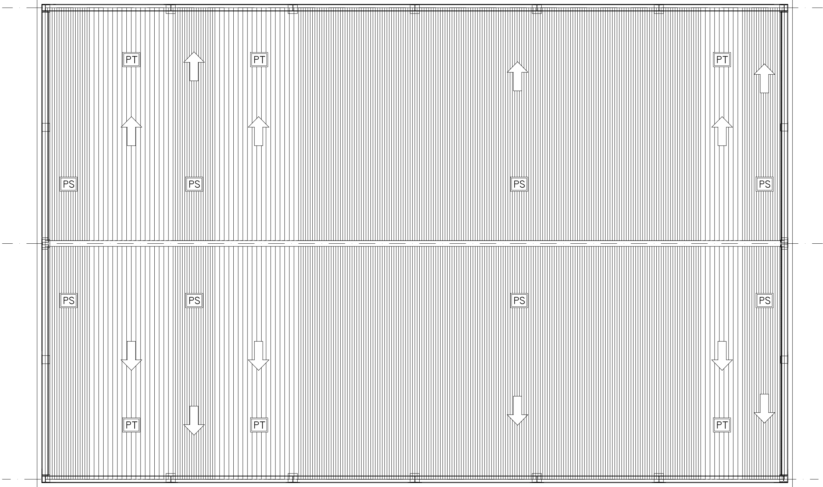
PLANTA DE CUBIERTA
