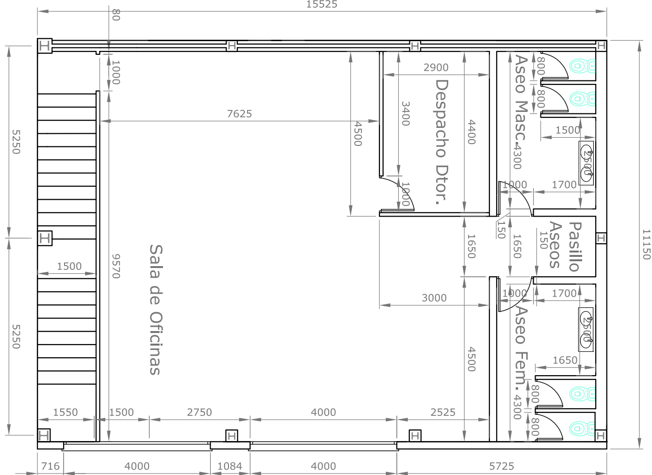
PLANTA PRIMERA
